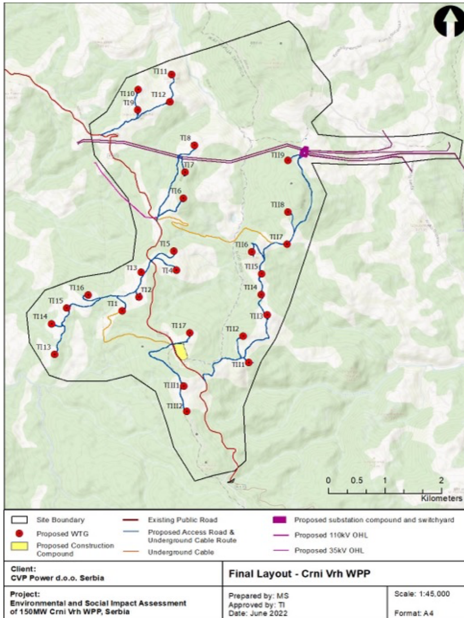
Slika 2 – Finalne pozicije turbina VE Crni Vrh
